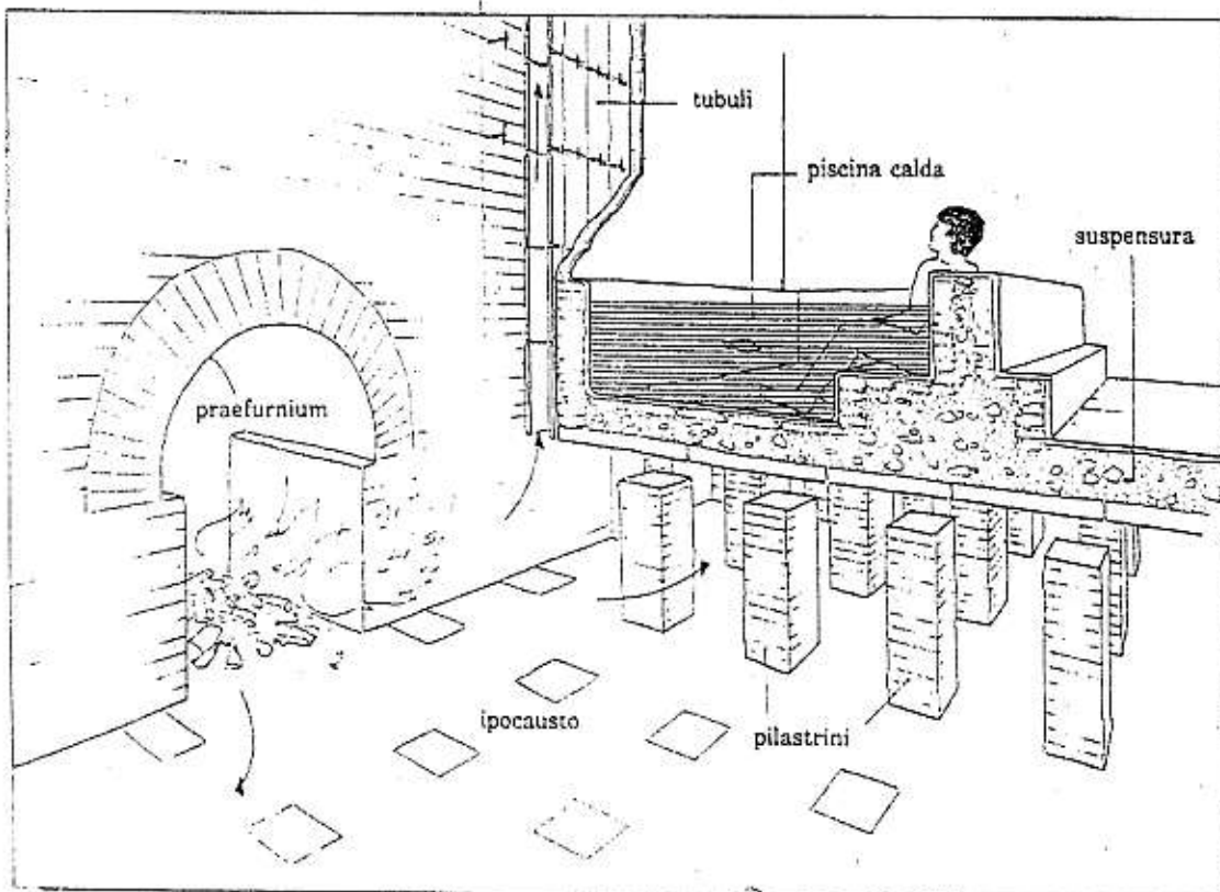
Funzionamento del riscaldamento del caldarium nelle Terme Centrali a Pompei. JPA
