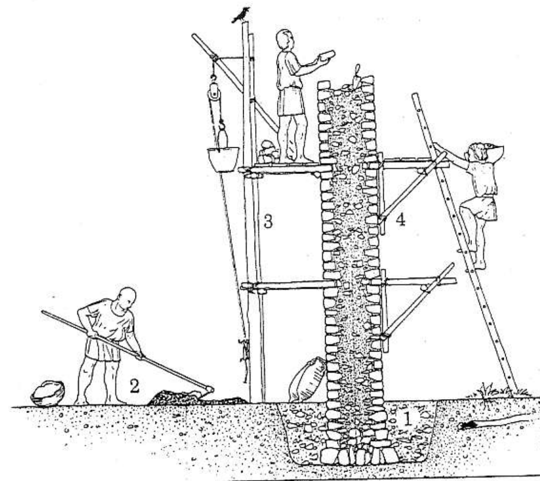
Costruzione di un muro. Riepilogo delle fasi di lavoro del cantiere: 1) trincea di fondazione; 2) preparazione della malta; 3) impalcatura a incastro con candele o antenne; 4) impalcatura a incastro a sbalzo. JPA
