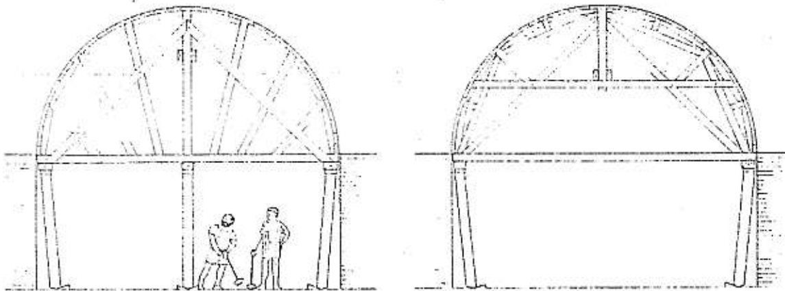
CENTINE PER VOLTE A BOTTE
