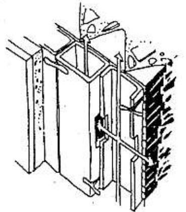
FUNZIONAMENTO TUBI IN COTTO PER IPOCAUSTO
