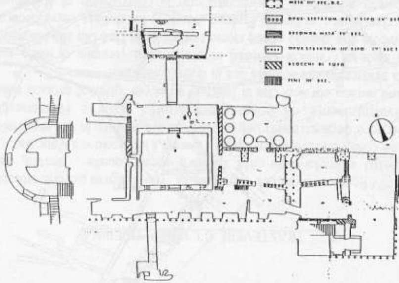
Pianta degli ambienti sotterranei di S. Cecilia
